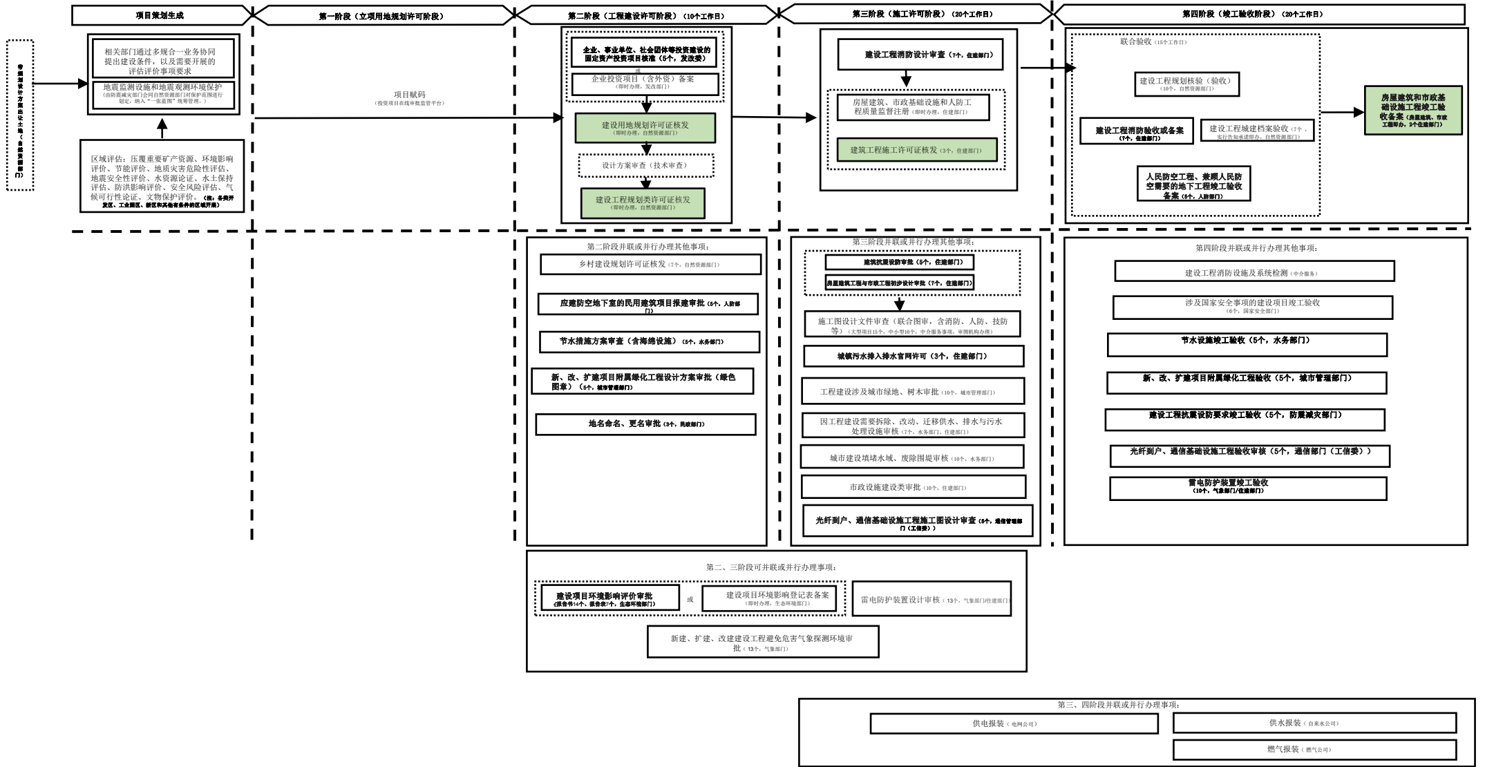
图6：昆明市工程建设项目审批流程图（社会投资带方案出让土地类建设项目）50天
